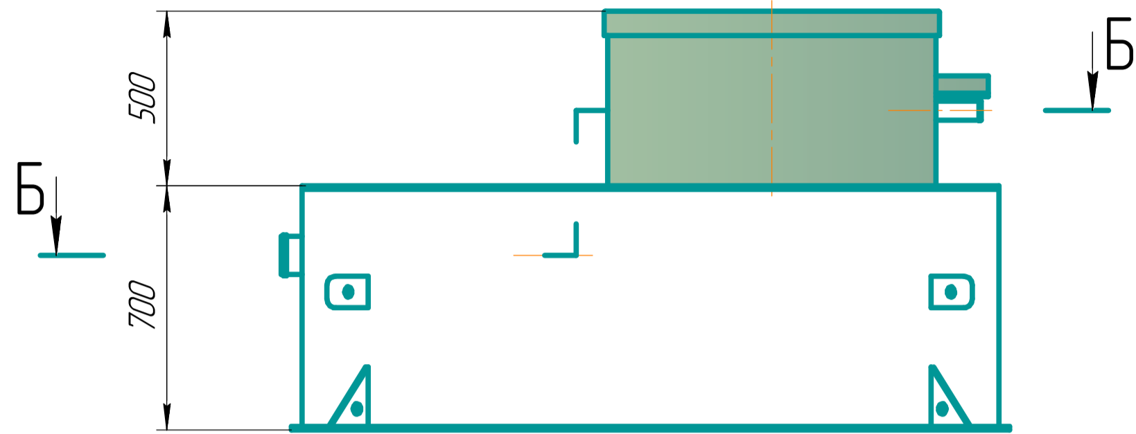
Вид спереди
